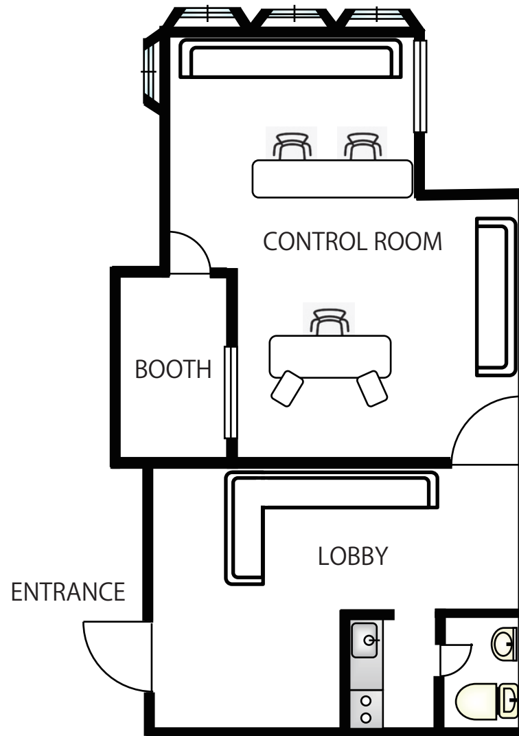
平面図
